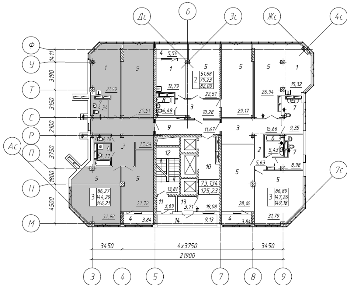
План квартиры № XX, отметка +XX, оси X-X, X-X
