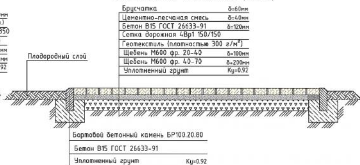
ПОКРЫТИЕ НА ОТМОСТКАХ (Тun 4)
