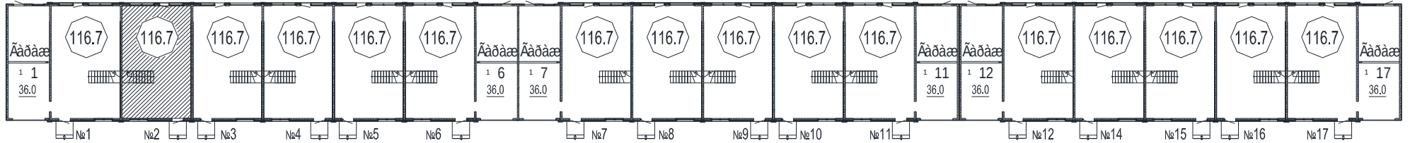
План 1 этажа
