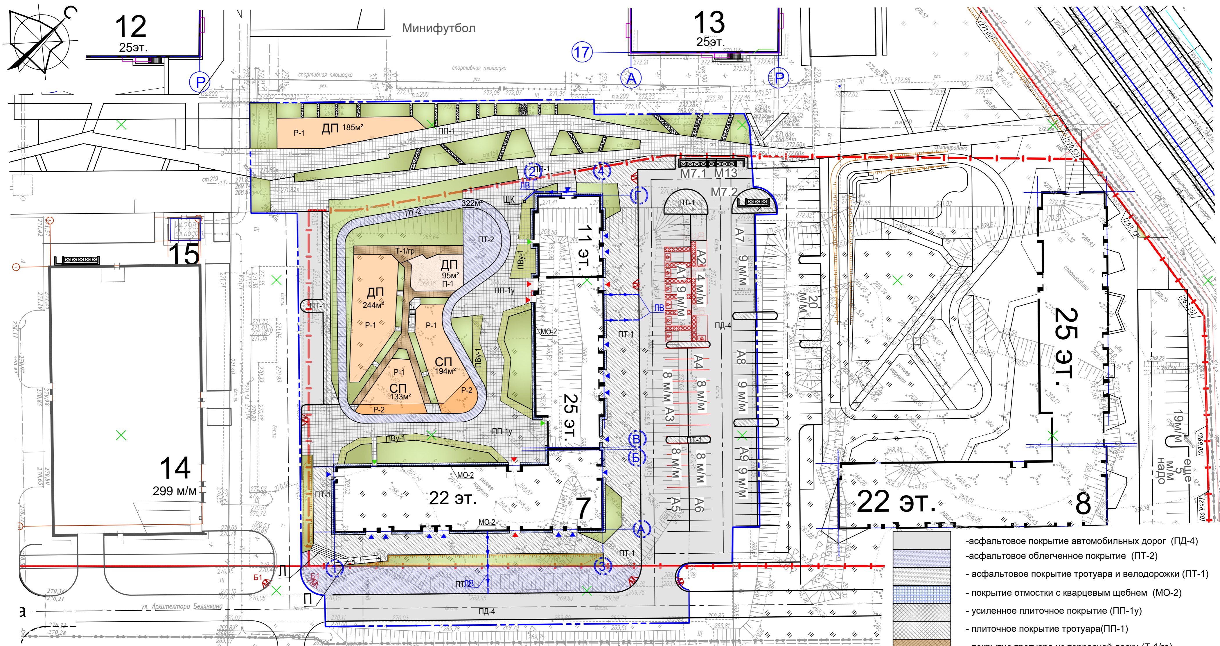
ЭКСПЛИКАЦИЯ ЗДАНИЙ И СООРУЖЕНИЙ
