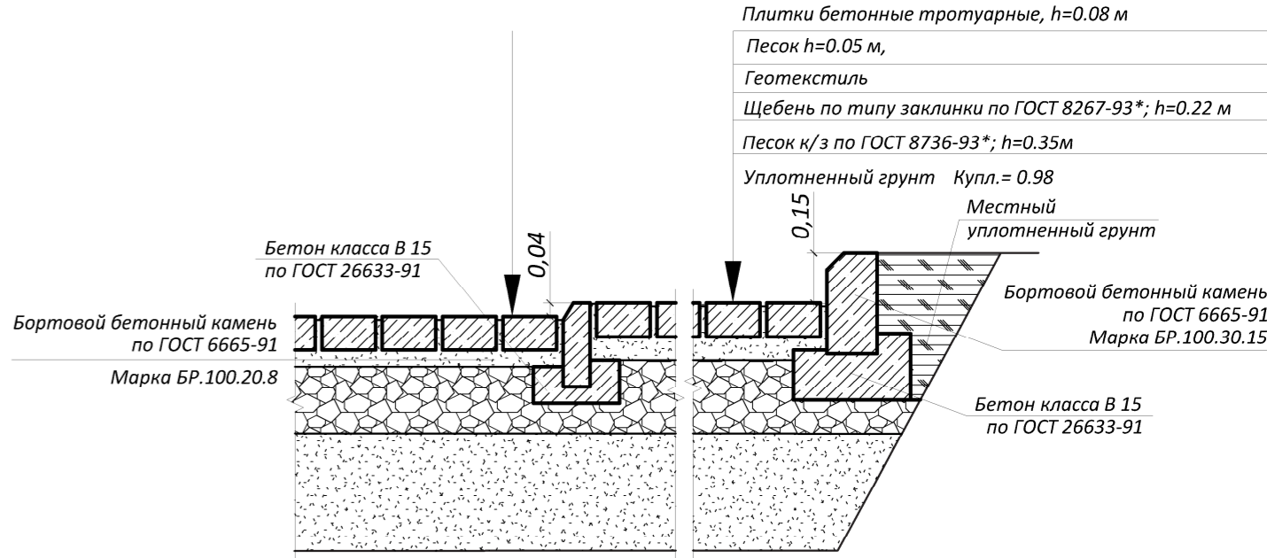
Проезд с мощением плиткой (тип 1)* Парковка с мощением плиткой (тип 2)*
