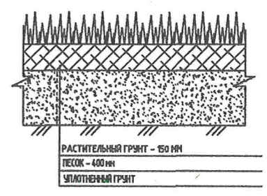
Деталь устройства усиленного газона
