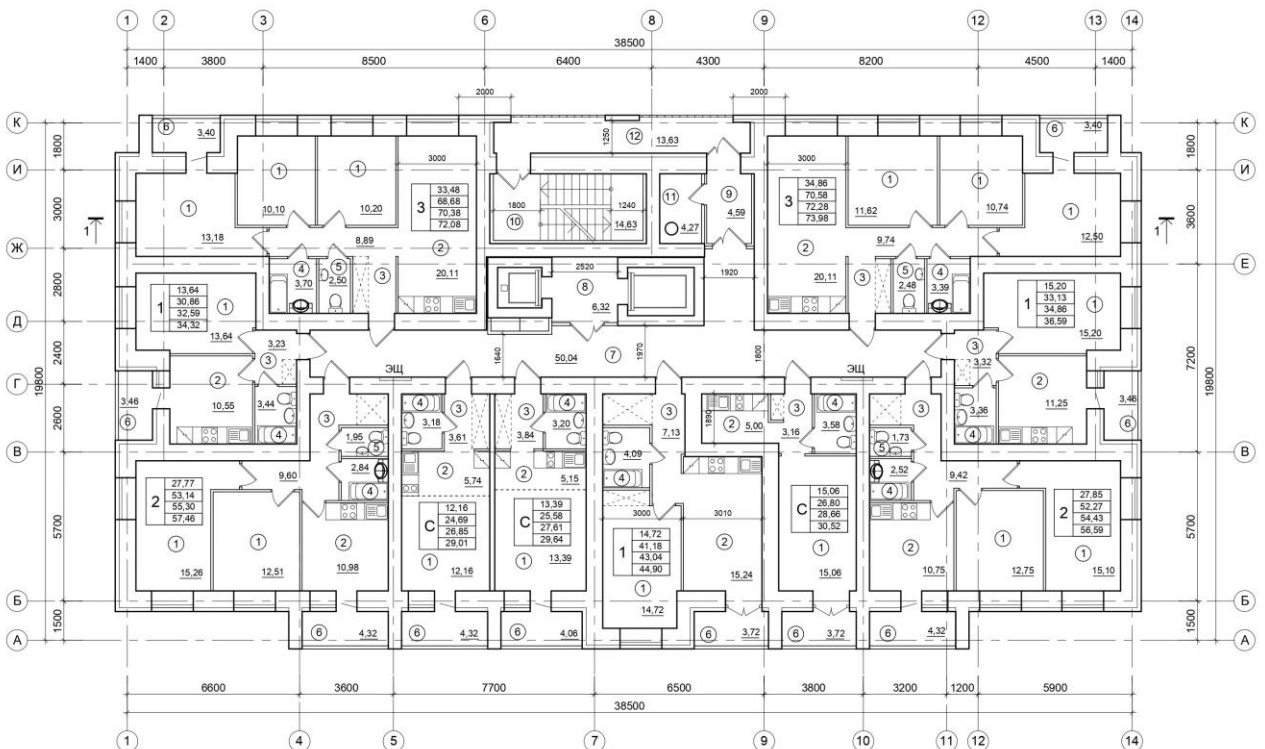
План 2-4 этажей
