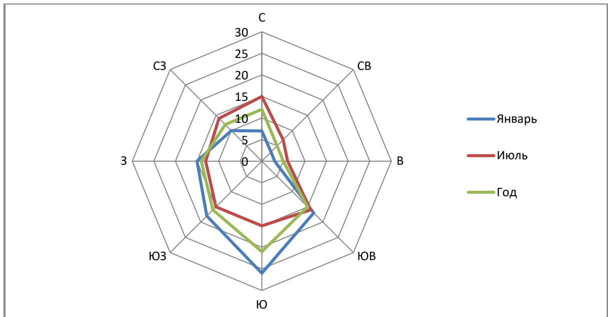
Рис. 9. Роза ветров, МС г. Кострома
