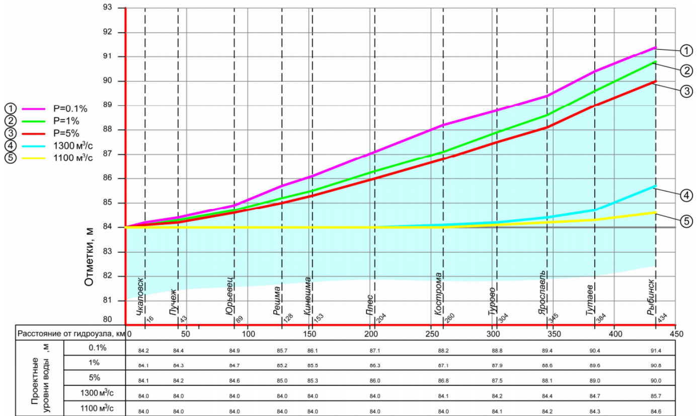
Рисунок Е.1. Расчетные кривые свободной поверхности Горьковского водохранилища
