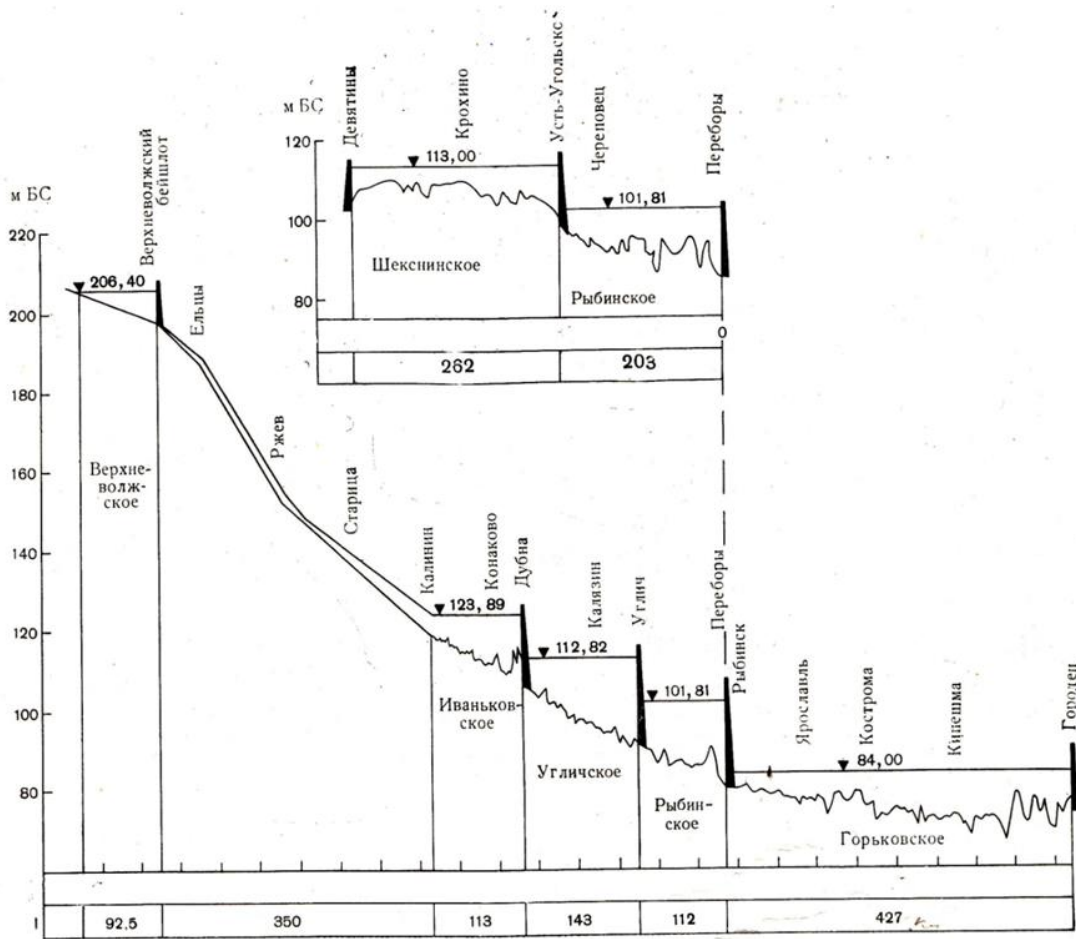
Рис. 7. Схема каскада верхневолжских водохранилищ
