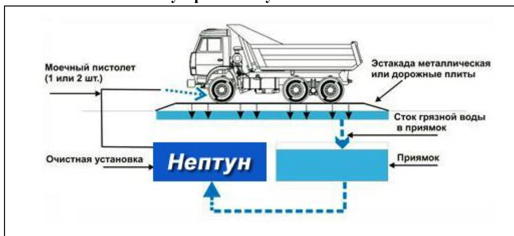
Схема устройства пункта мойки колёс
