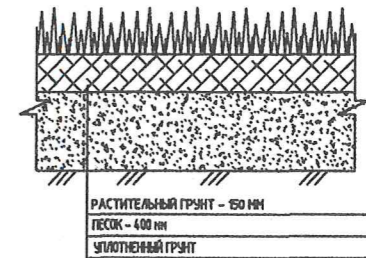
Деталь устройства усиленного газона
