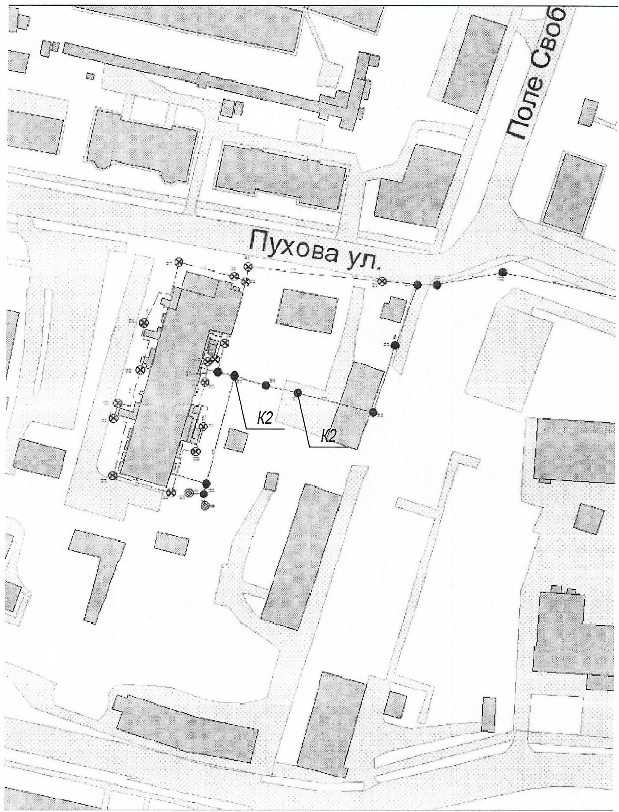
K2- точки подключения к уличной сети поверхностного стока
