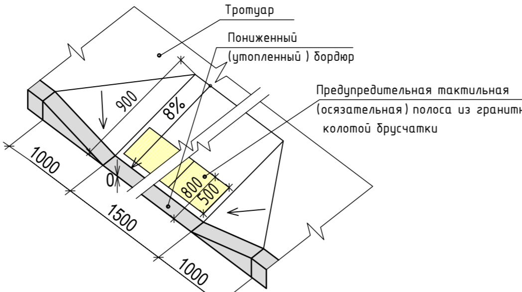
ДЕТАЛЬ УСТРОЙСТВА Пониженного бордюра И2
