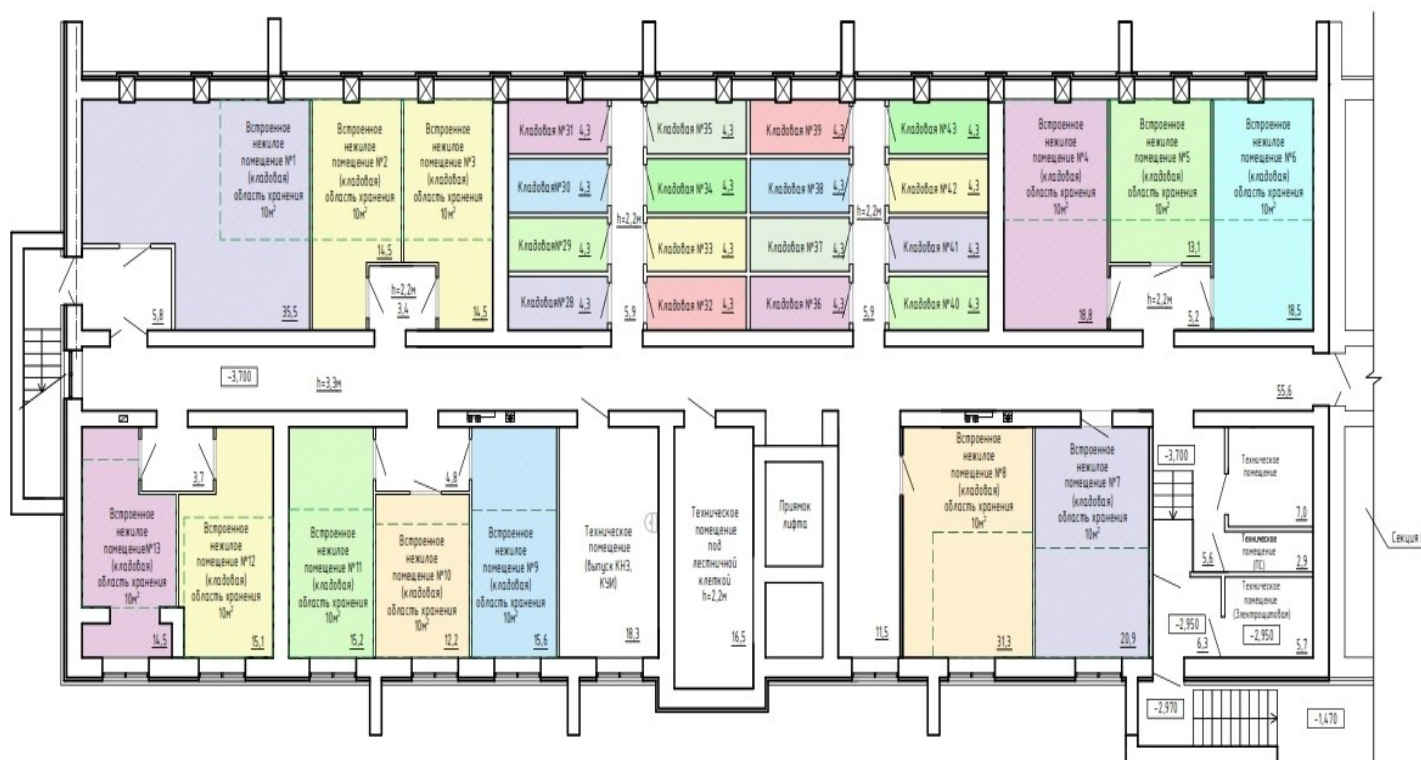
План подвала. Секция №1
