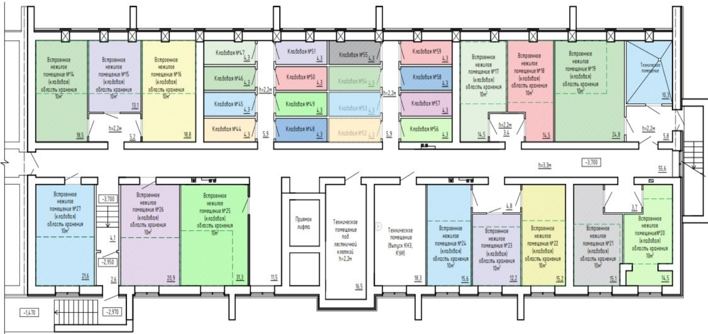
План подвала. Секция №2
