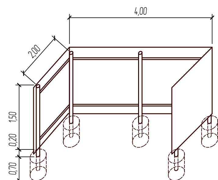
Эскиз ограждения хозяйственной площадки
