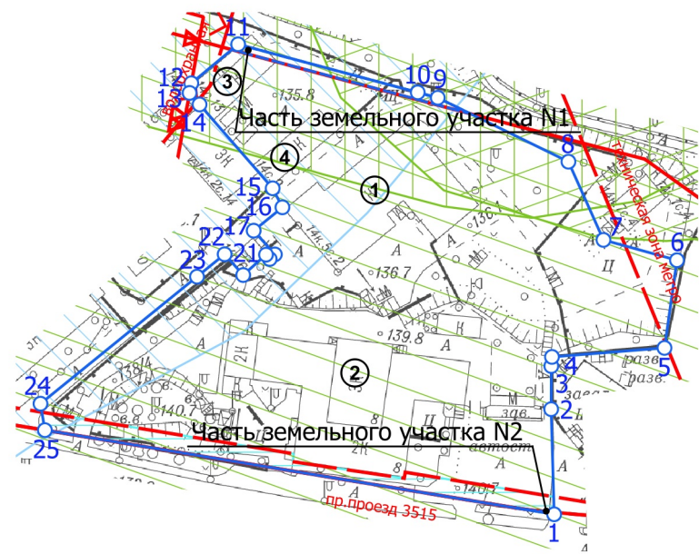
Ситуационный план
