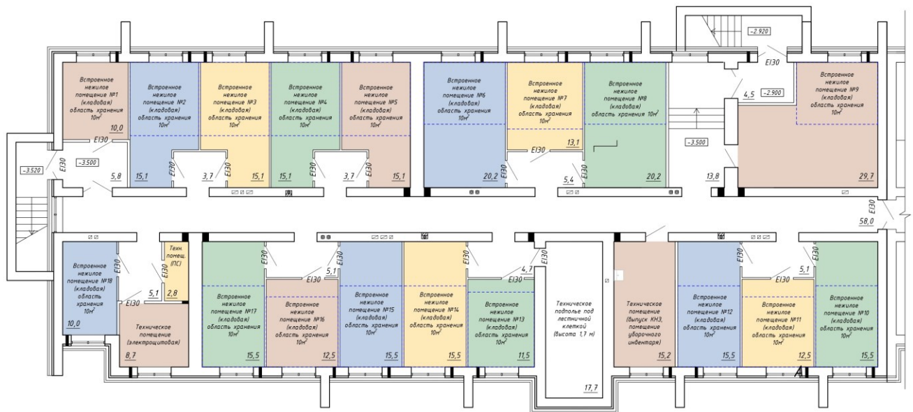
План подвального этажа (секция 1)
