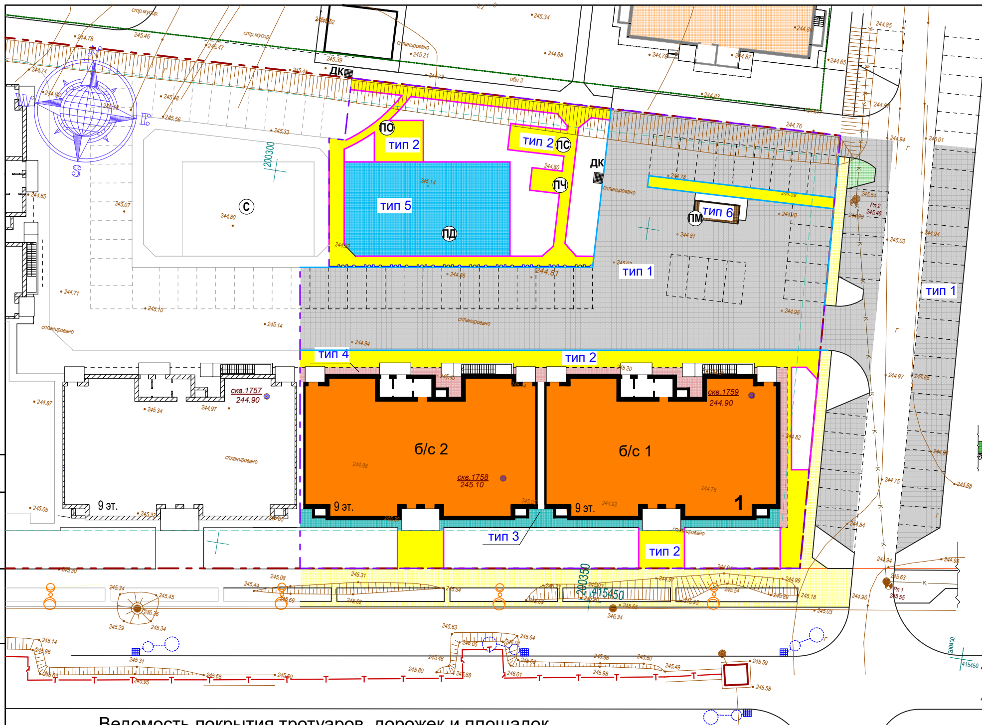
Ведомость покрытия тротуаров, дорожек и площадок
