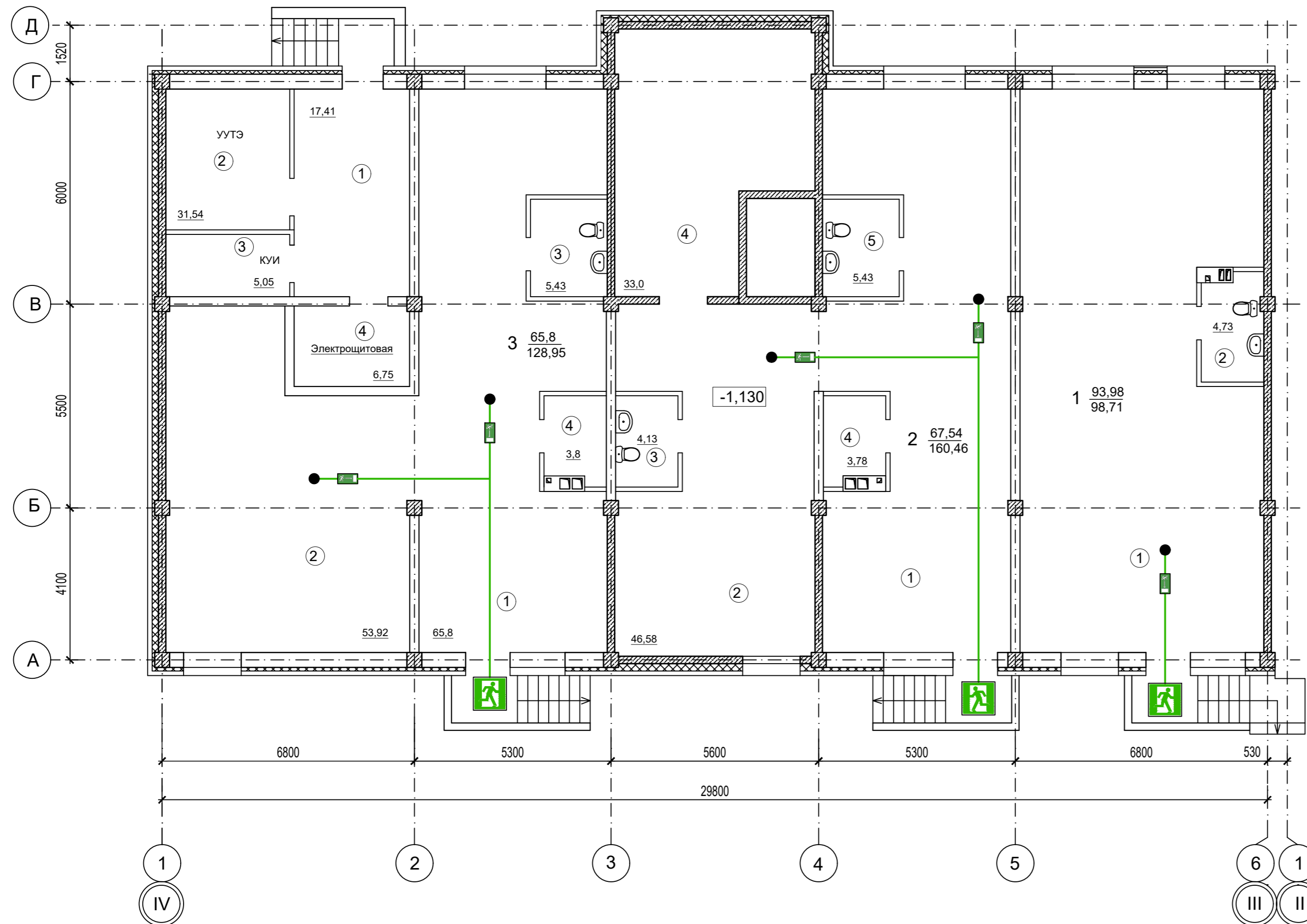
Компоновочная схема
