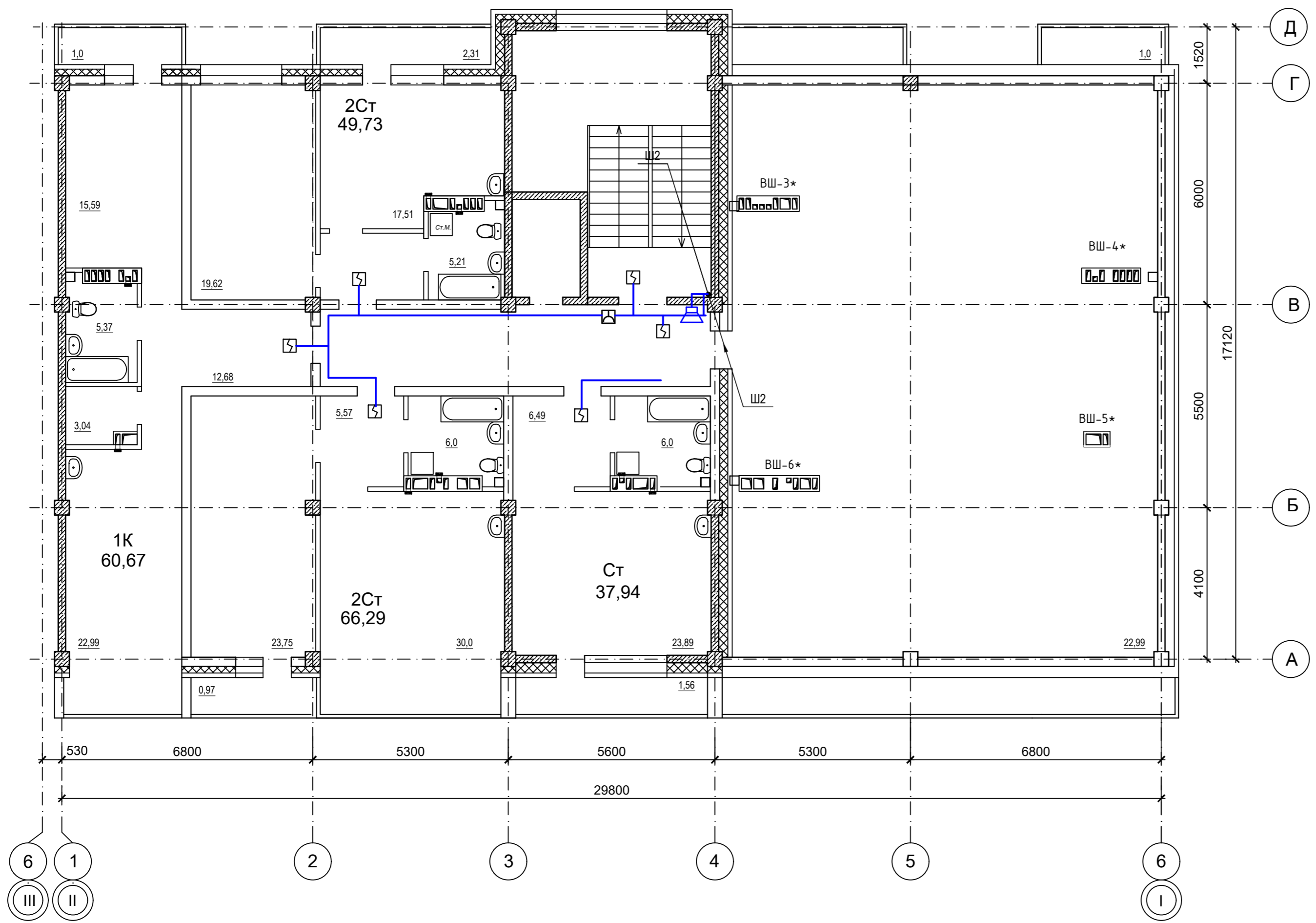
Компоновочная схема
