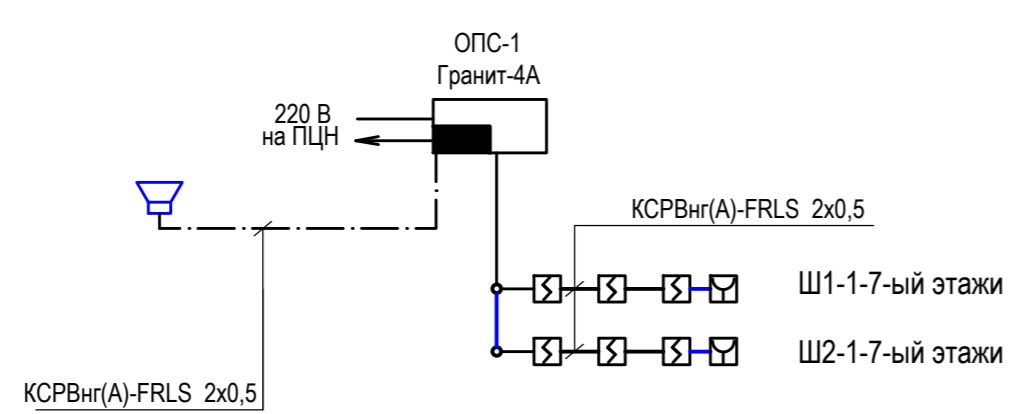
Структурная схема
