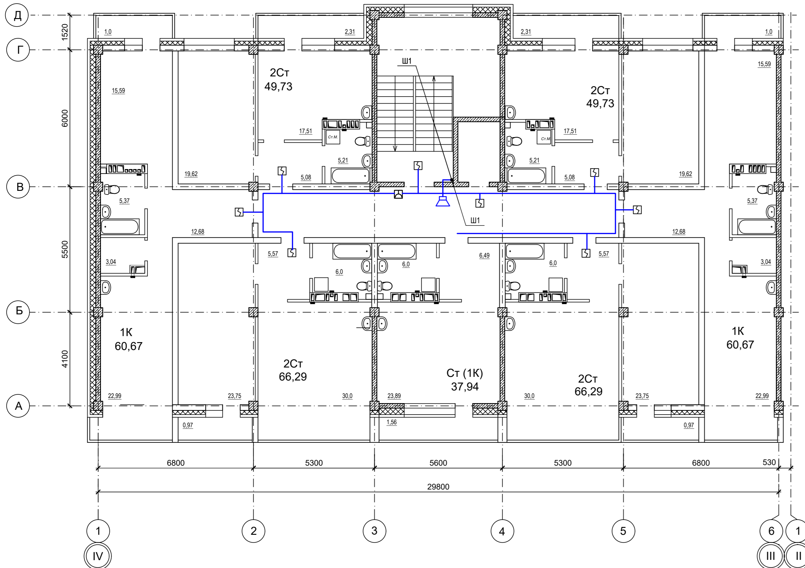
Компоновочная схема
