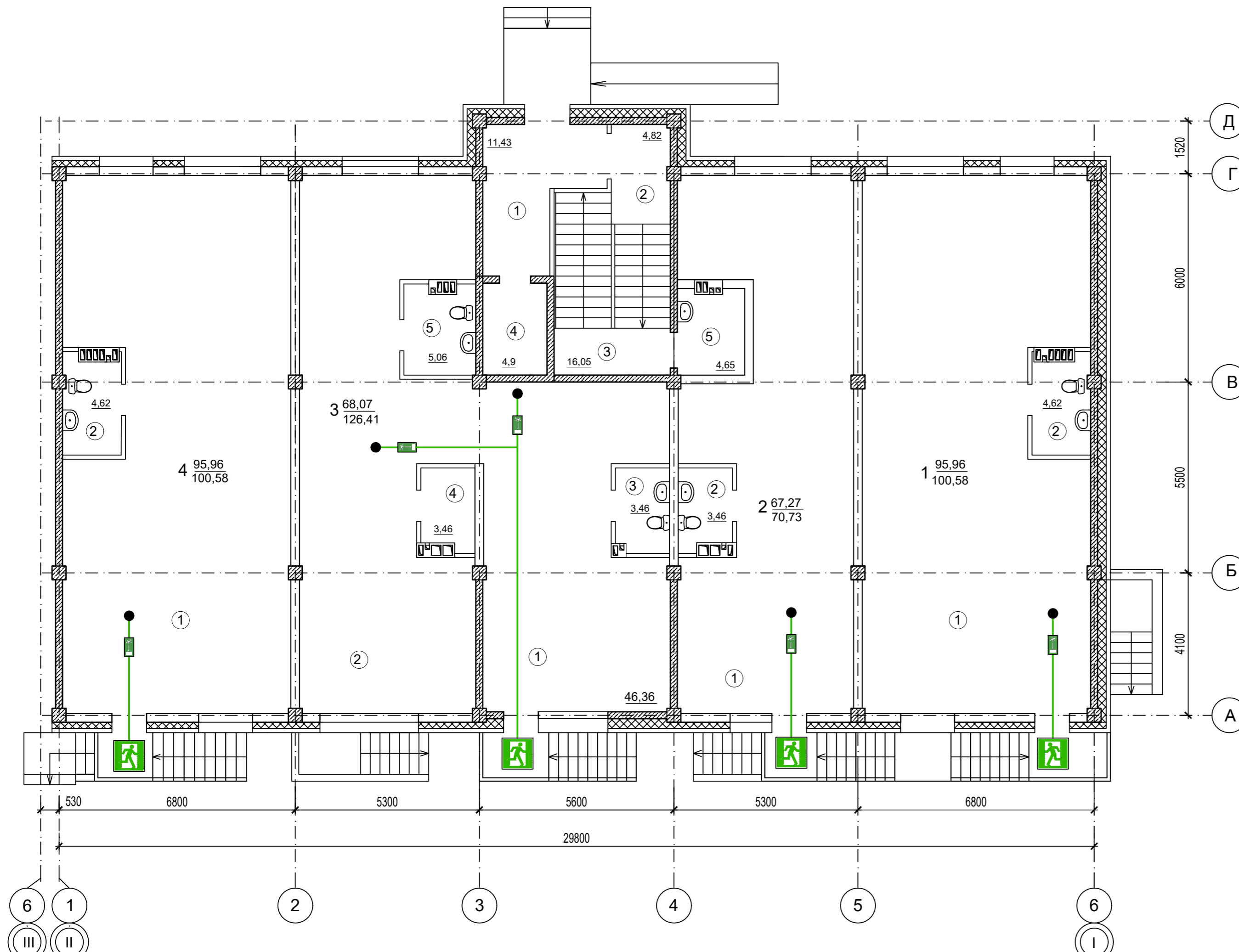
Компоновочная схема
