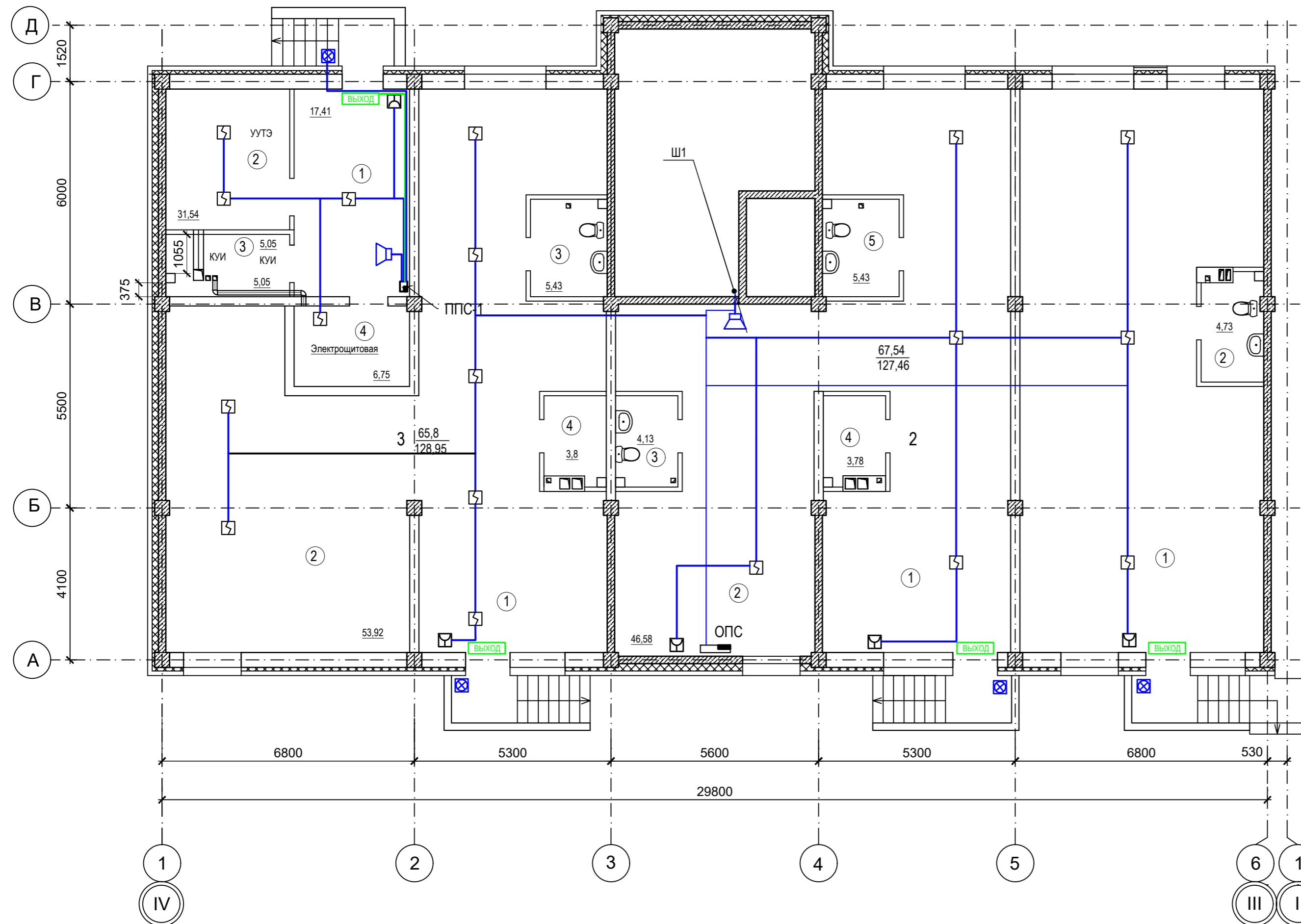
Компоновочная схема
