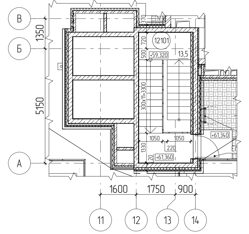
Фрагмент плана выхода на кровлю в осях 11-14/A-B
