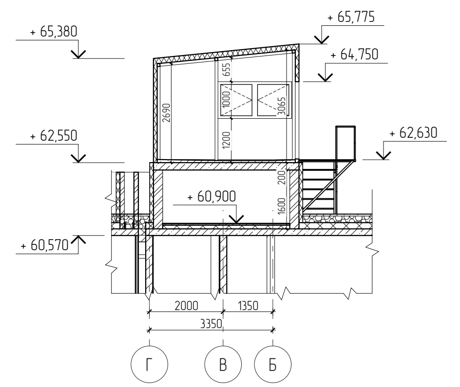
Разрез 5-5
