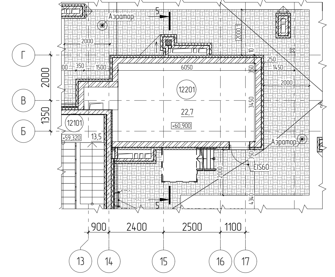
План пространства для прокладки коммуникаций в осях 13-17/Б-Г
