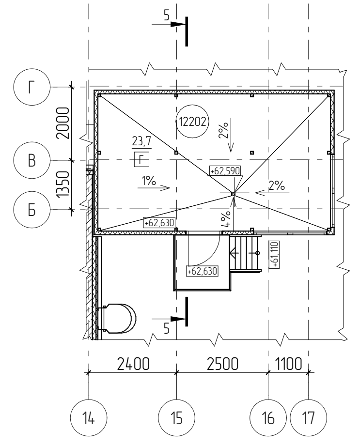
План котельной на отметке +62,630
