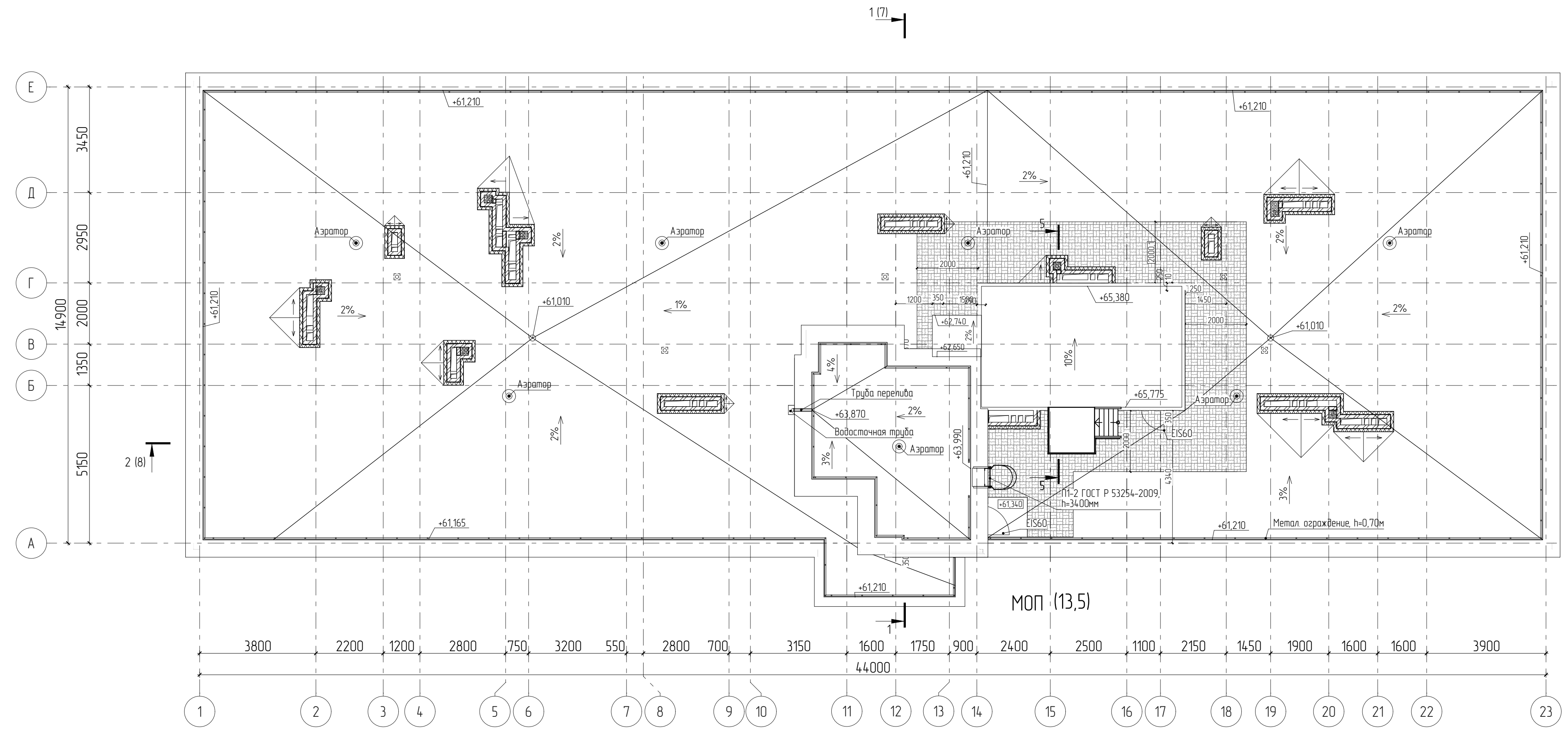
План кровли 1 (7)
