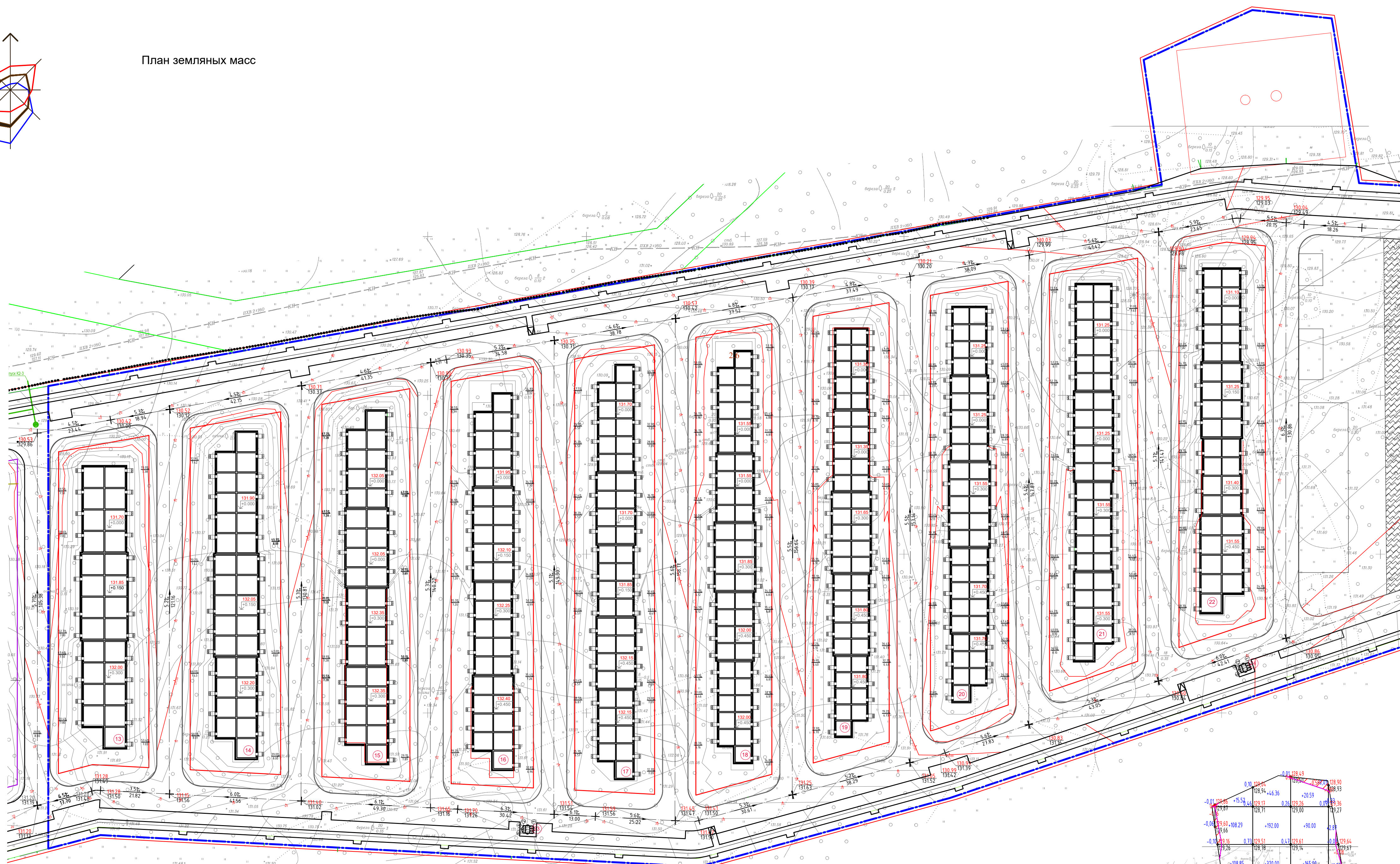
План земляных масс
