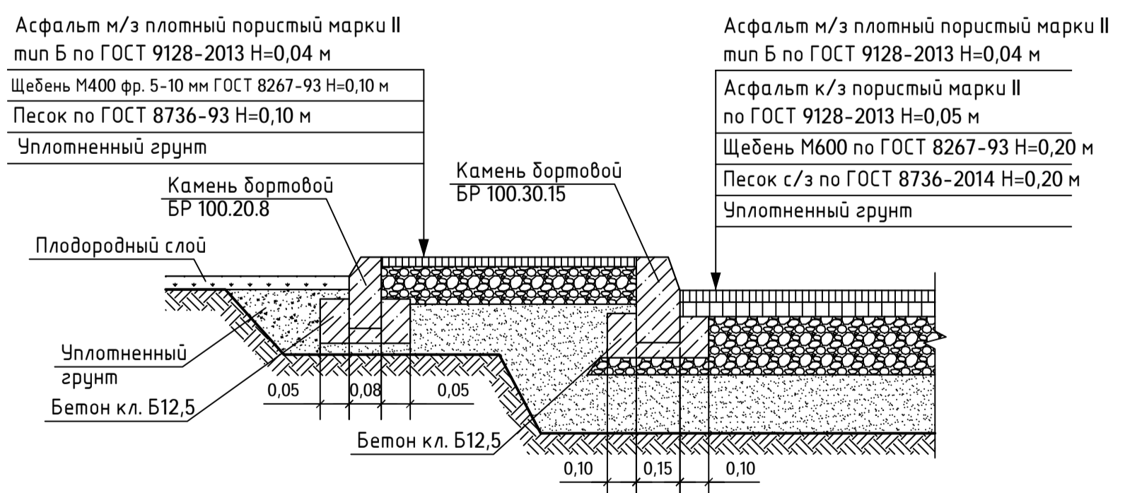
УЗЕЛ СОПРЯЖЕНИЯ ПРОЕЗДА (ТИП I) С ТРОТУАРОМ (ТИП II)
