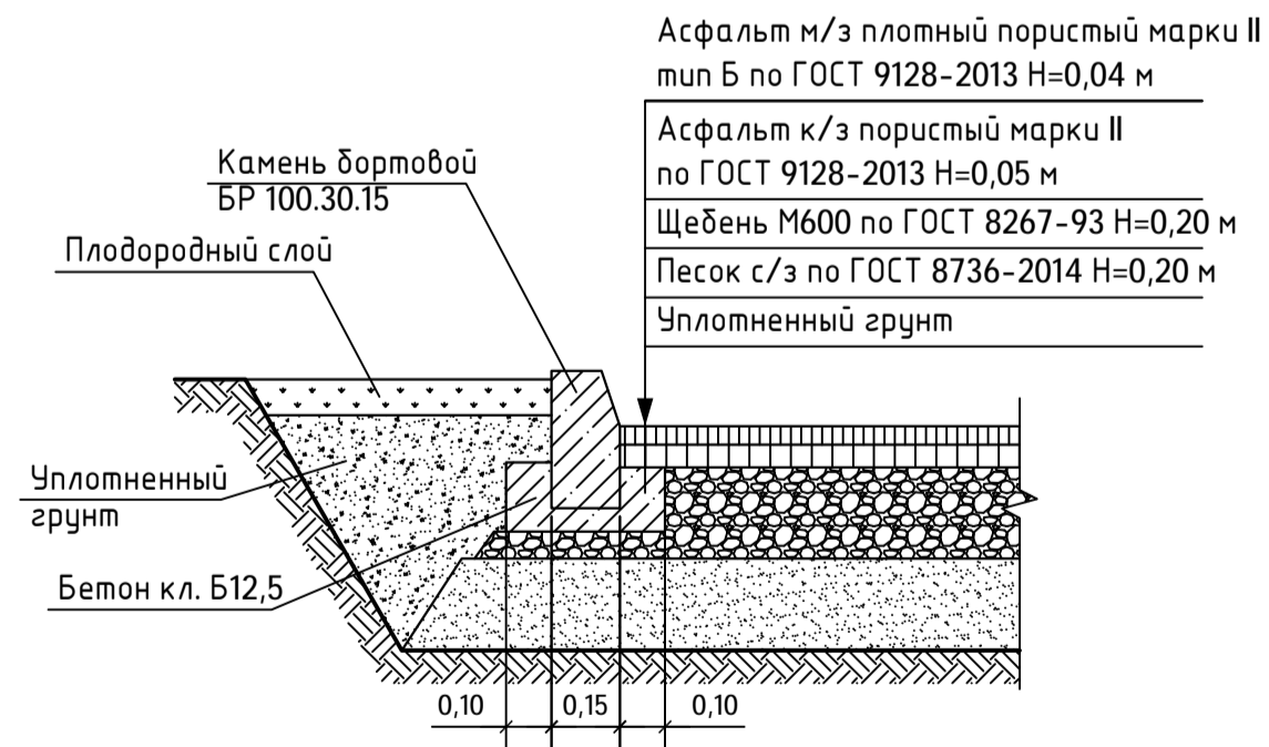
УЗЕЛ СОПРЯЖЕНИЯ ПРОЕЗДА (ТИП I) С ГАЗОНОМ
