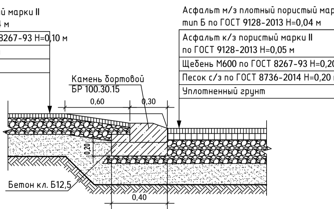
УЗЕЛ ПЕРЕСЕЧЕНИЯ ПРОЕЗДА С ТРОТУАРОМ ДЛЯ МГН (УЗЕЛ А)
