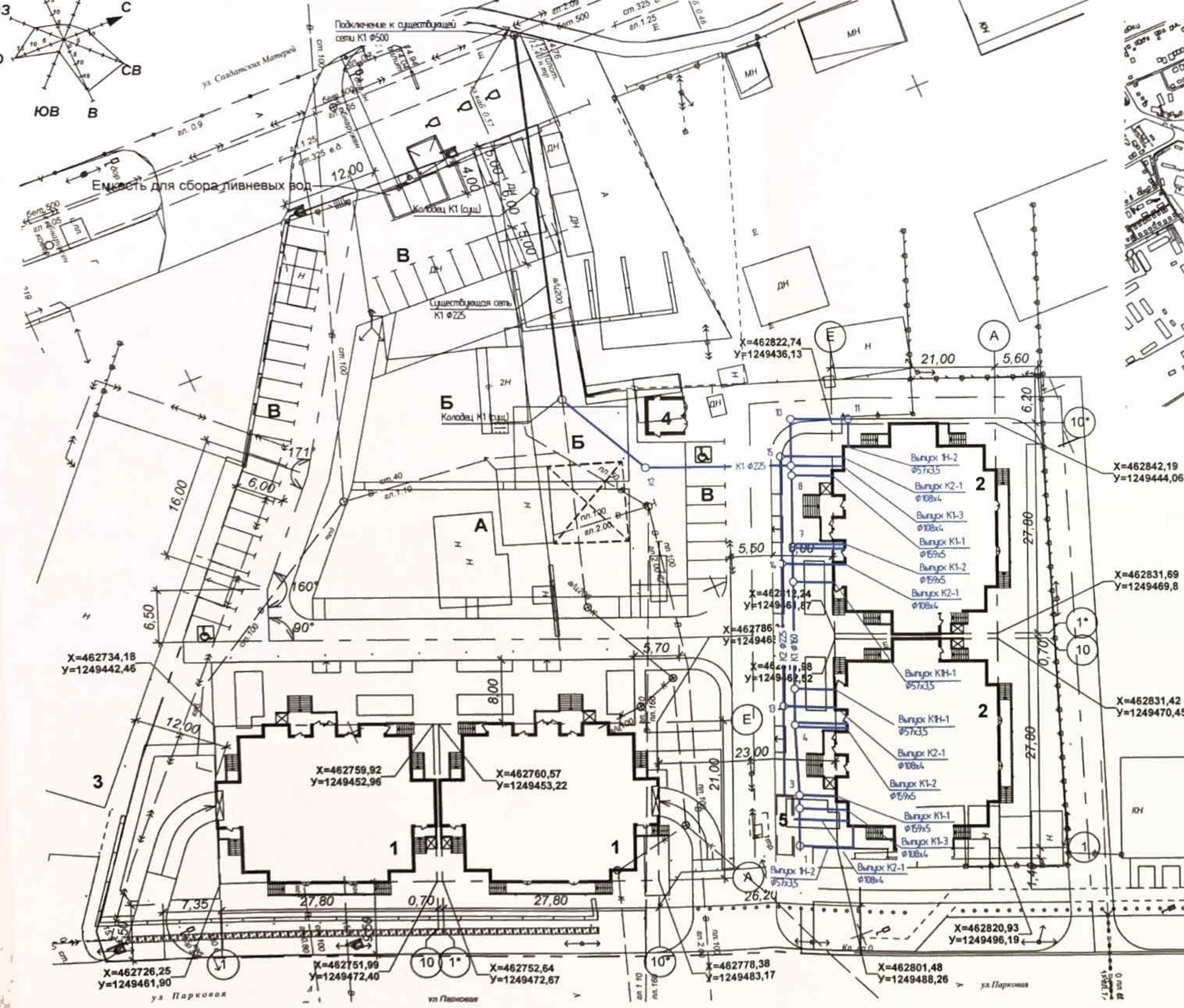
РАЗБИВОЧНЫЙ ПЛАН. М 1:500.
