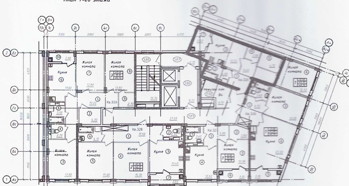
План 7-го этажа
