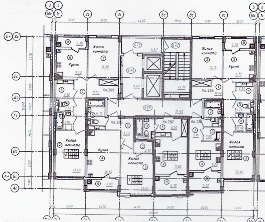
План 10-го этажа
