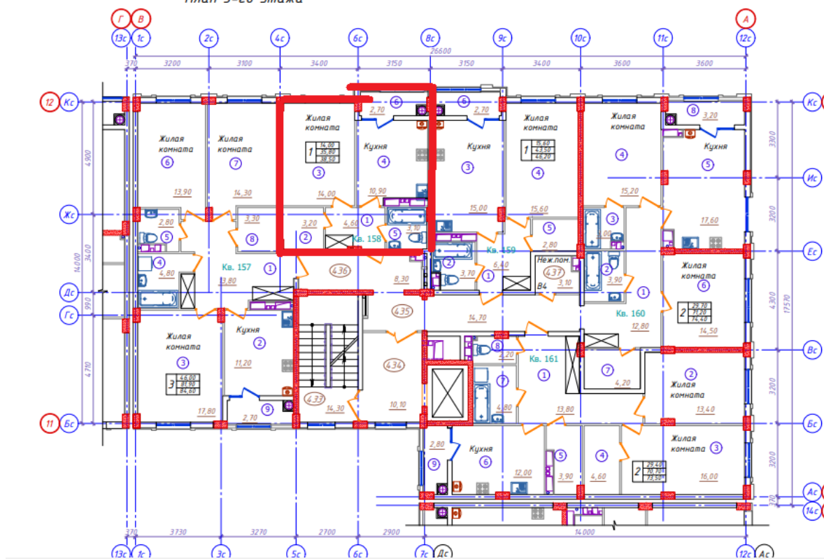
План 3-го этажа
