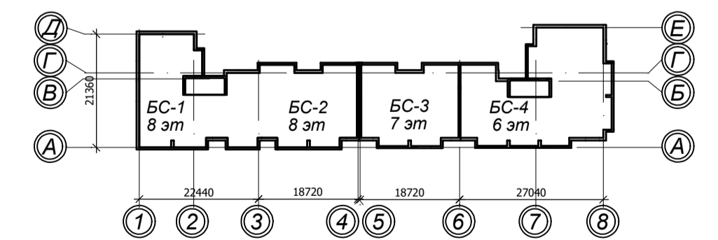
КОМПОНОВочная СХЕМА
