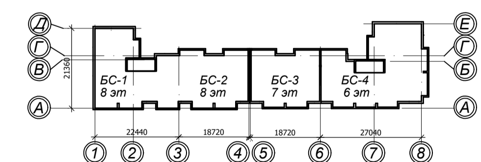
КОМПОНОВОЧНАЯ СХЕМА
