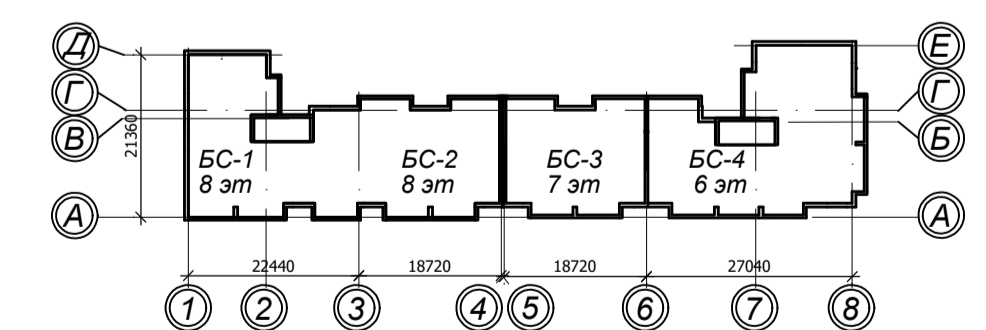
КОМПОЗОВАННАЯ СХЕМА
