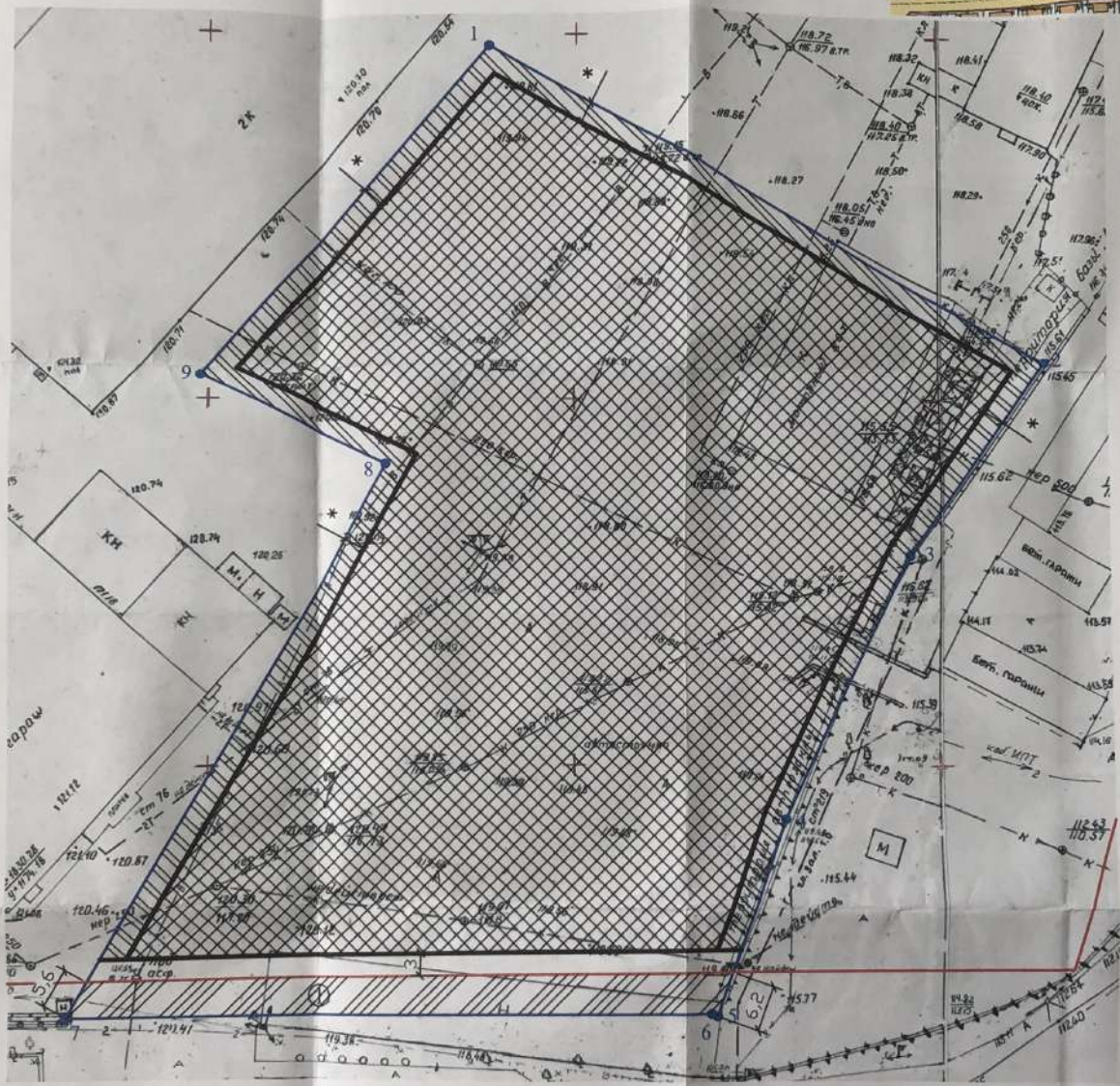
1. Чертеж градостроительного плана земельного участка
