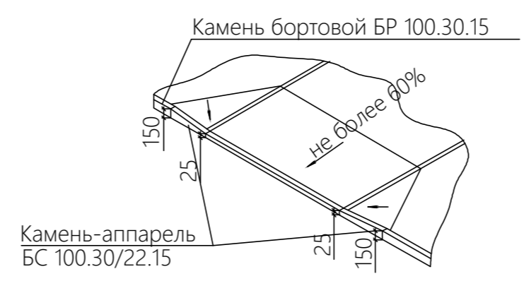
Узел понижения бортового камня
