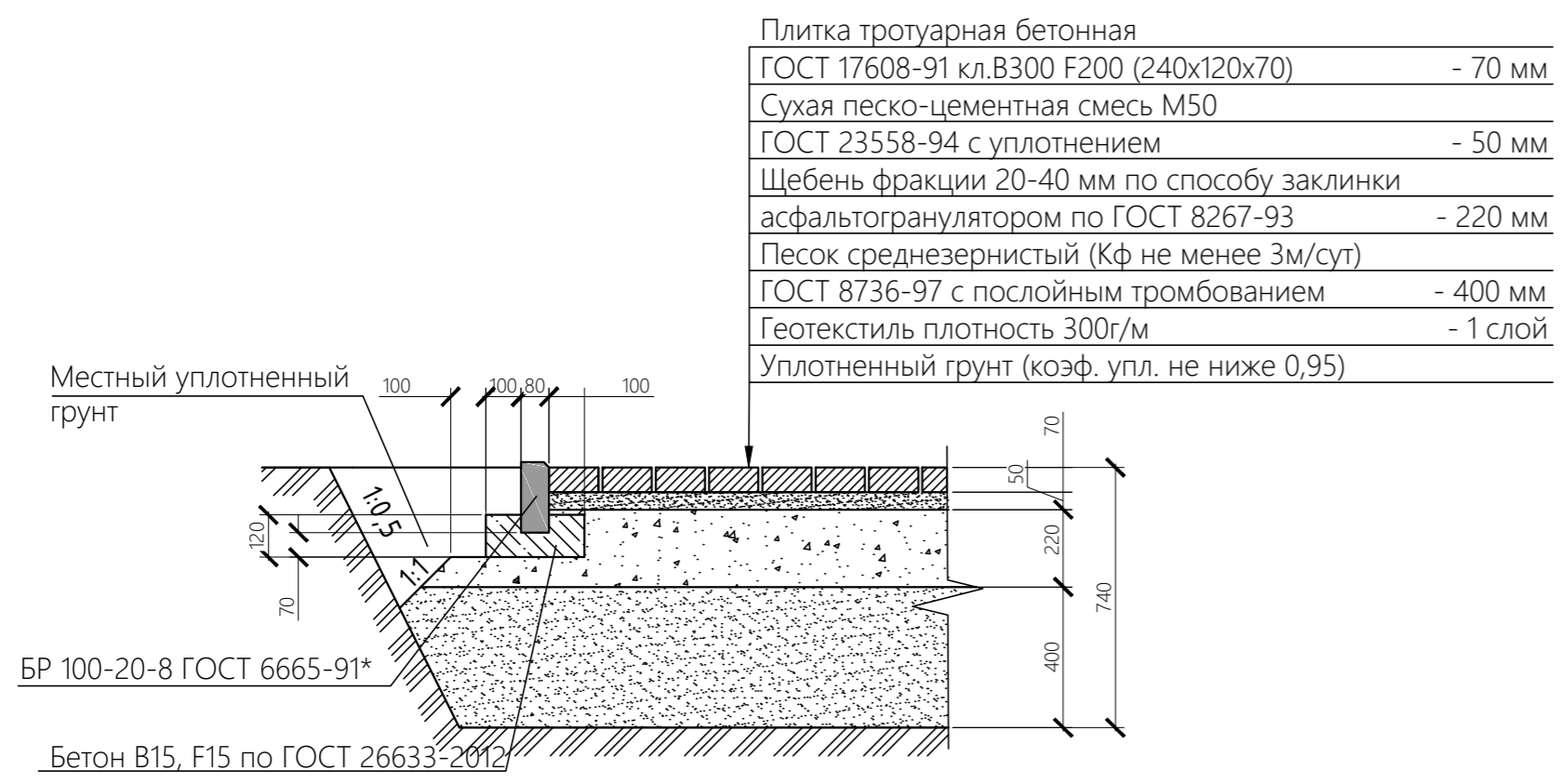
Тип 3 (тротуар с возможностью проезда пожарной машины)
