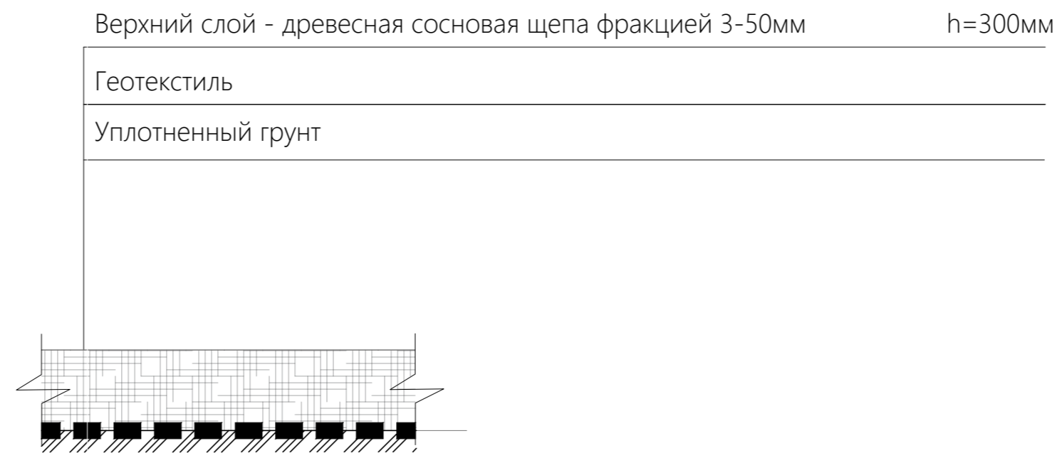
Тип 4 (покрытие детской площадки древесная щепа) (безопасная h_{\text{падения}}=3.0\text{м} )
