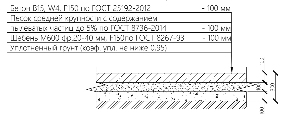
Тип 6 (бетонная площадка под контейнеры ТБО)
