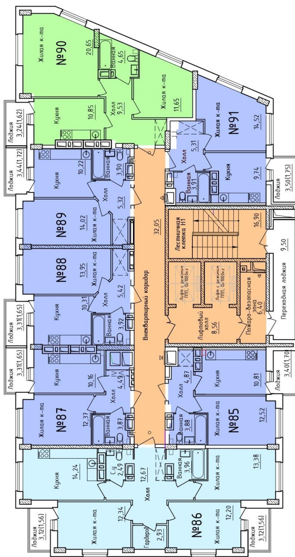
План 14-го этажа на отм. +39,600
