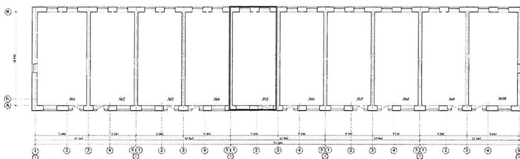
План планировки 2 этажа
