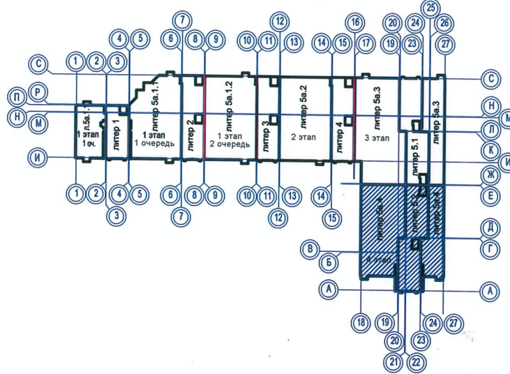
Компоновочная схема
