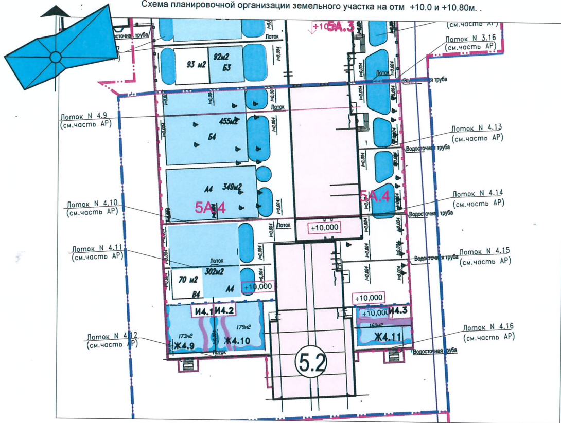
Схема планировочной организации земельного участка на отм +10.0 и +10.80м.
