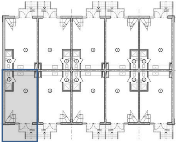
2 этаж
